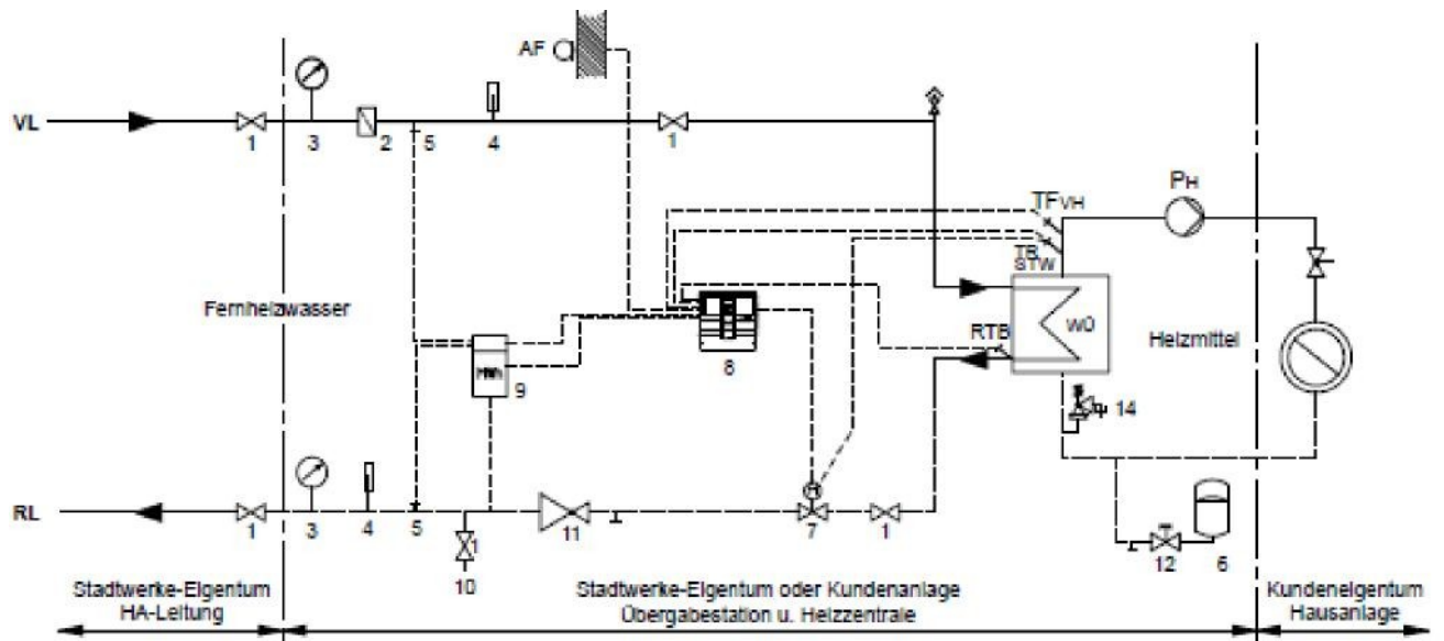
Abb. 2 Schaltschema
